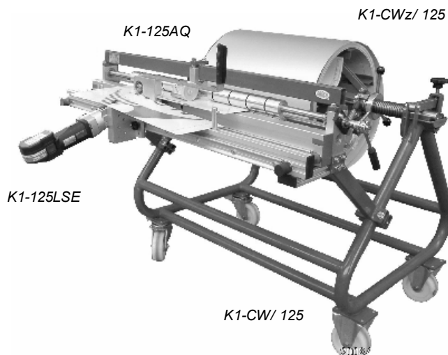
Coilwagen + Haspel K1-CW/ 125 met afrol en dwarsnijdinrichting K1-125AQ, Langsnijdinrichting K1-125LSE met accu metaalschaar AK 3514-2
